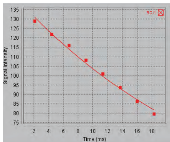
ABBILDUNG 4. T2Star-Kurve
