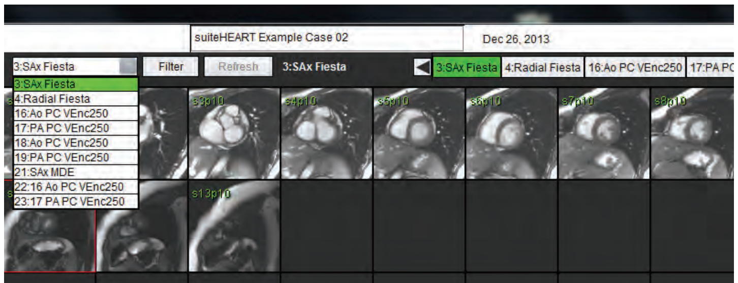
ABBILDUNG 2. Serien-Navigation
